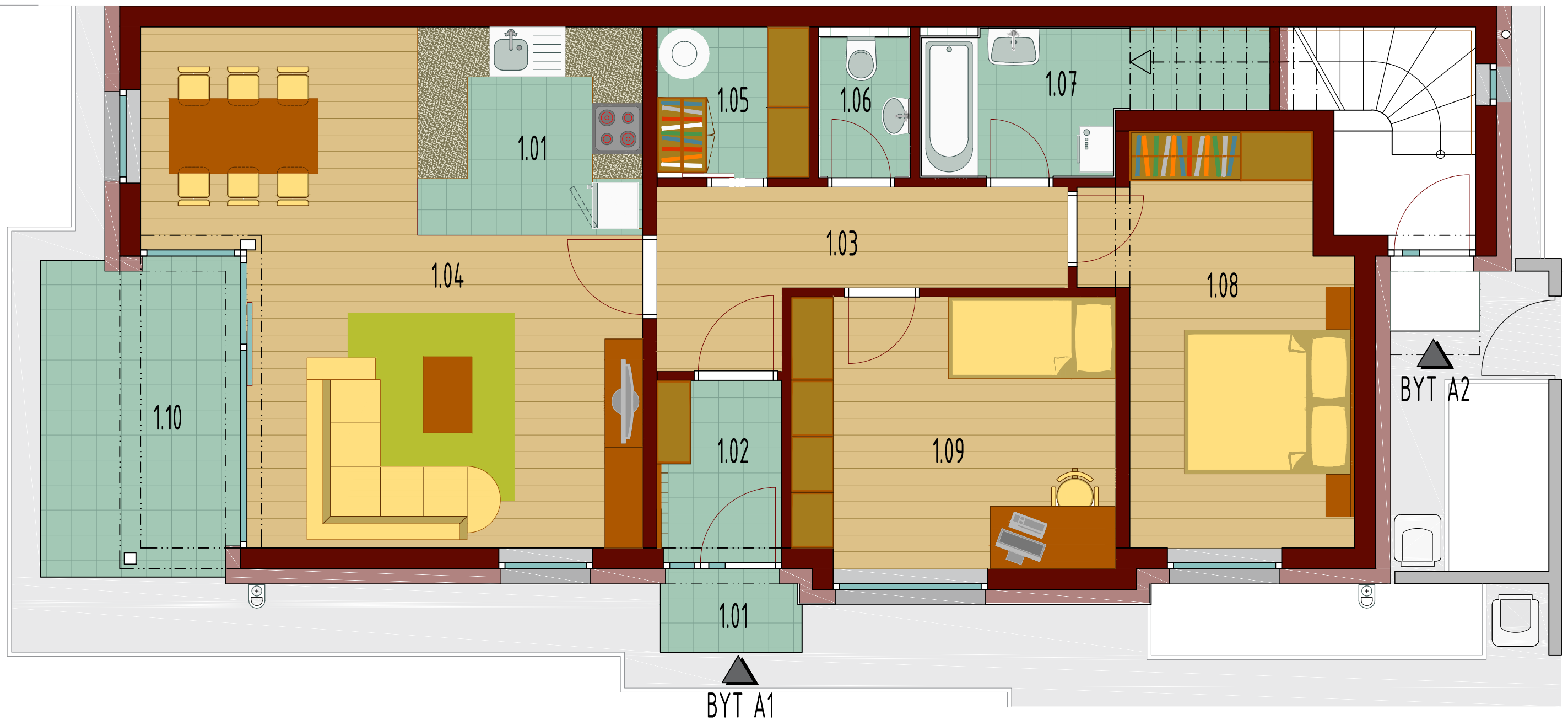
PÔDORYS 1.N.P.
