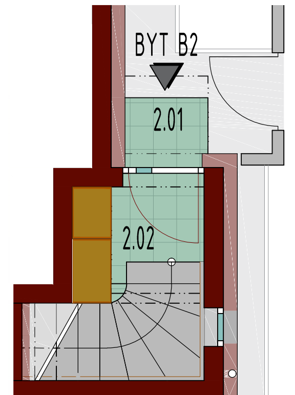
PÔDORYS 1.N.P.
