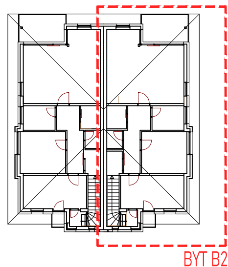
SCHÉMA 2.N.P.
